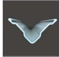
завальцованный край увеличивает жёсткость стойки
